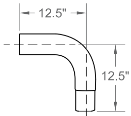
90° Elbow (P/N: E6)
