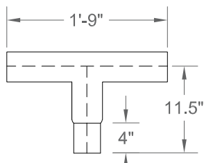
Tee (P/N: V-T or V-TI)
